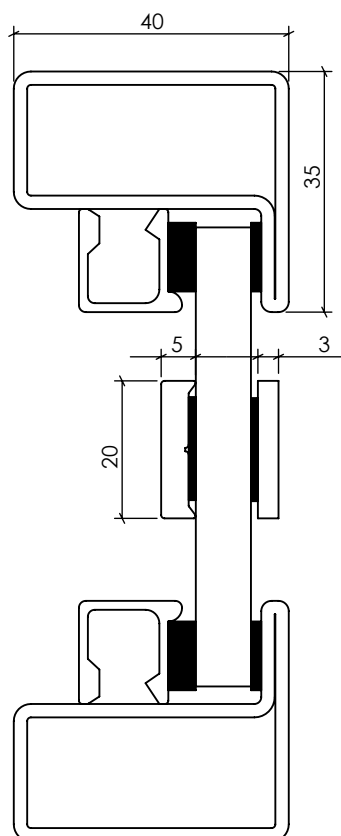
LOFT 35 SZPROS NAKLEJANY 20mm
