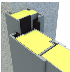
Przekrój: skrzydło/ościeżnica
