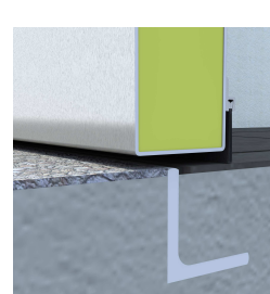
Przekrój: drzwi bezprogowe Kątownik 50/50/6mm↓
