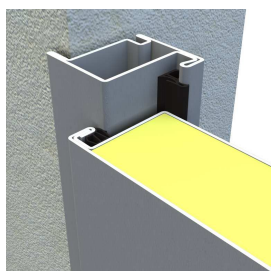
Przekrój: skrzydło/ościeżnica
