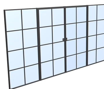
Propozycja drzwi dwuskrzydłowych z klamką LOFT i z witryną
